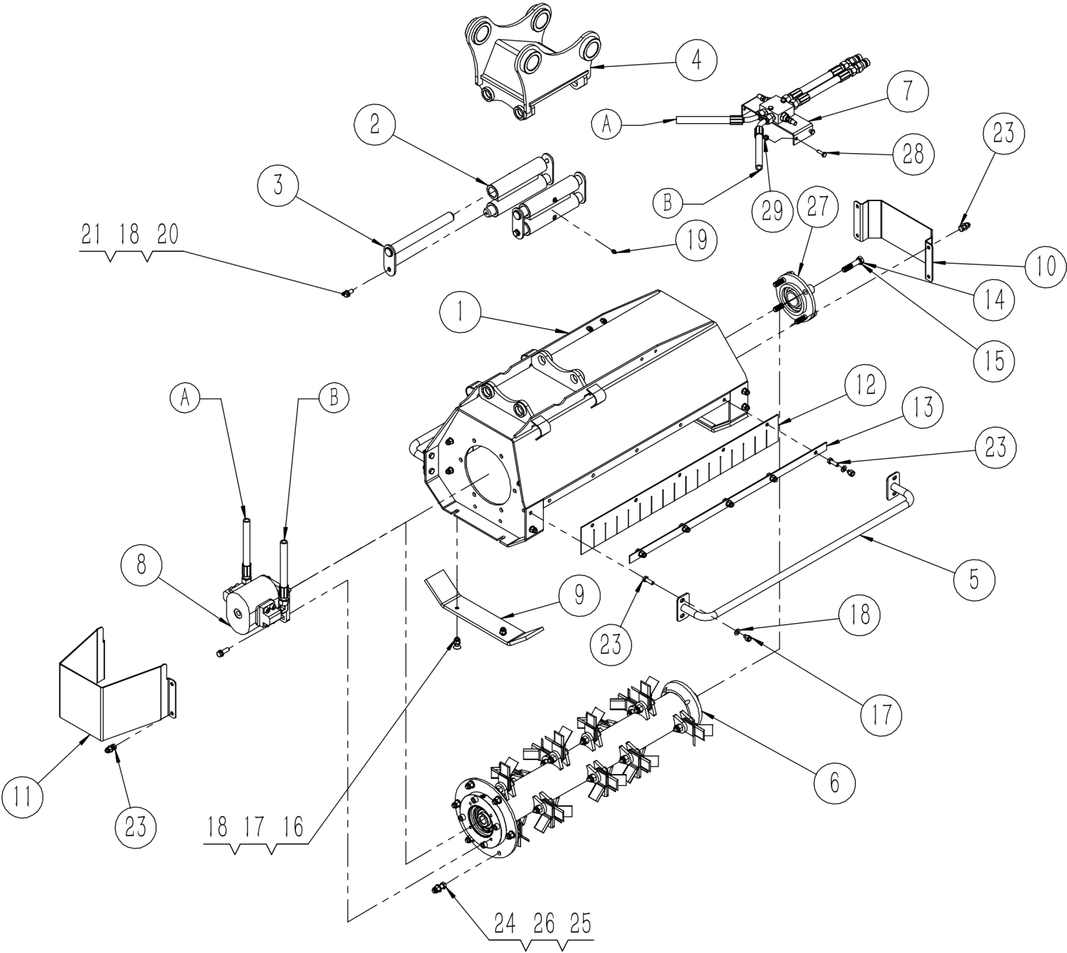
大正工業ショベルモア分解図 本体部分(2024/09/30)
