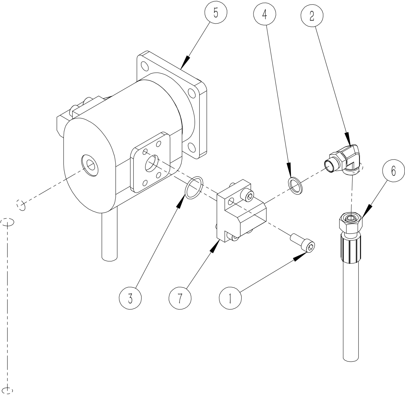
大正工業ショベルモア分解図 油圧モーター部分(2024/09/30)
