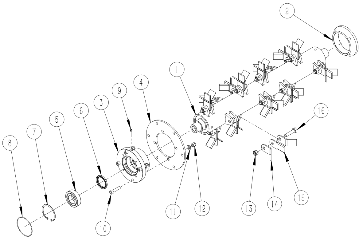
大正工業ショベルモア分解図 カッターシャフト部分(2024/09/30)
